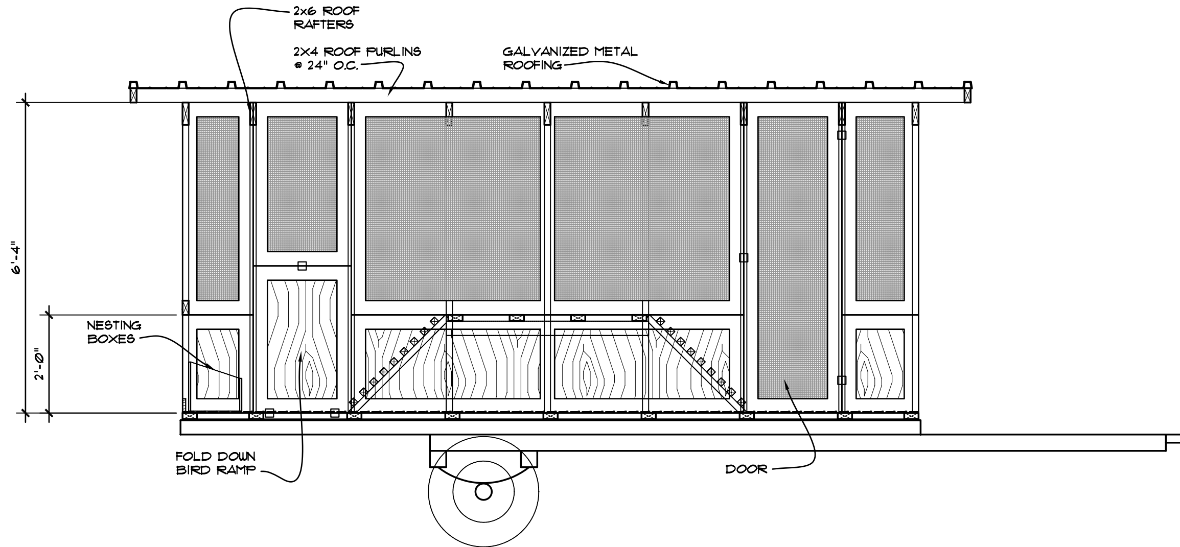
ELEVATION - 1 SCALE: 1/2" = 1'-0"
